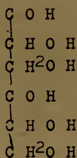
Aldehido glicérico
