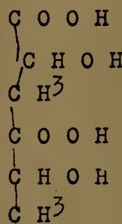
Acido láctico
