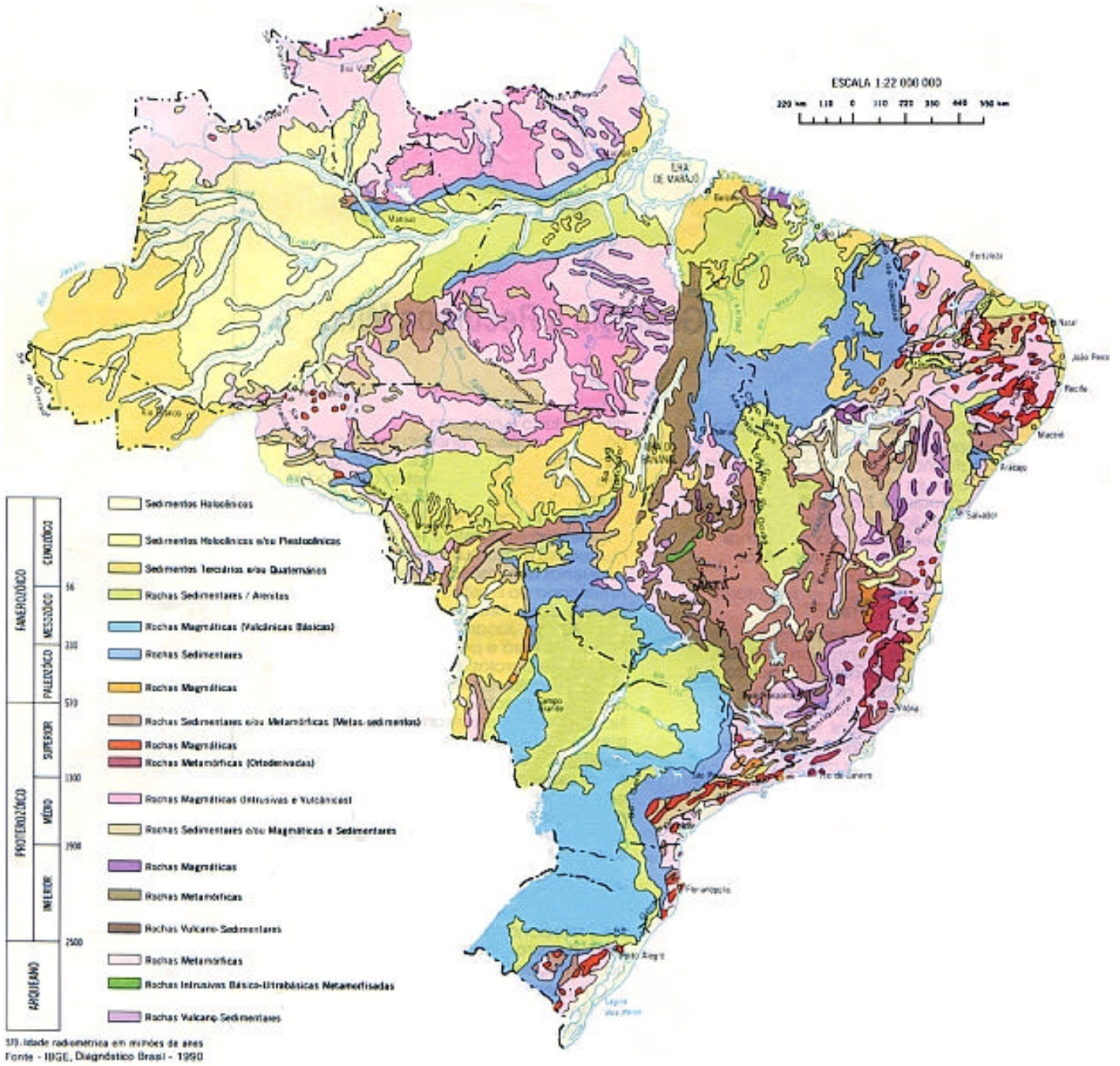
Mapa 1.15 Geologia
