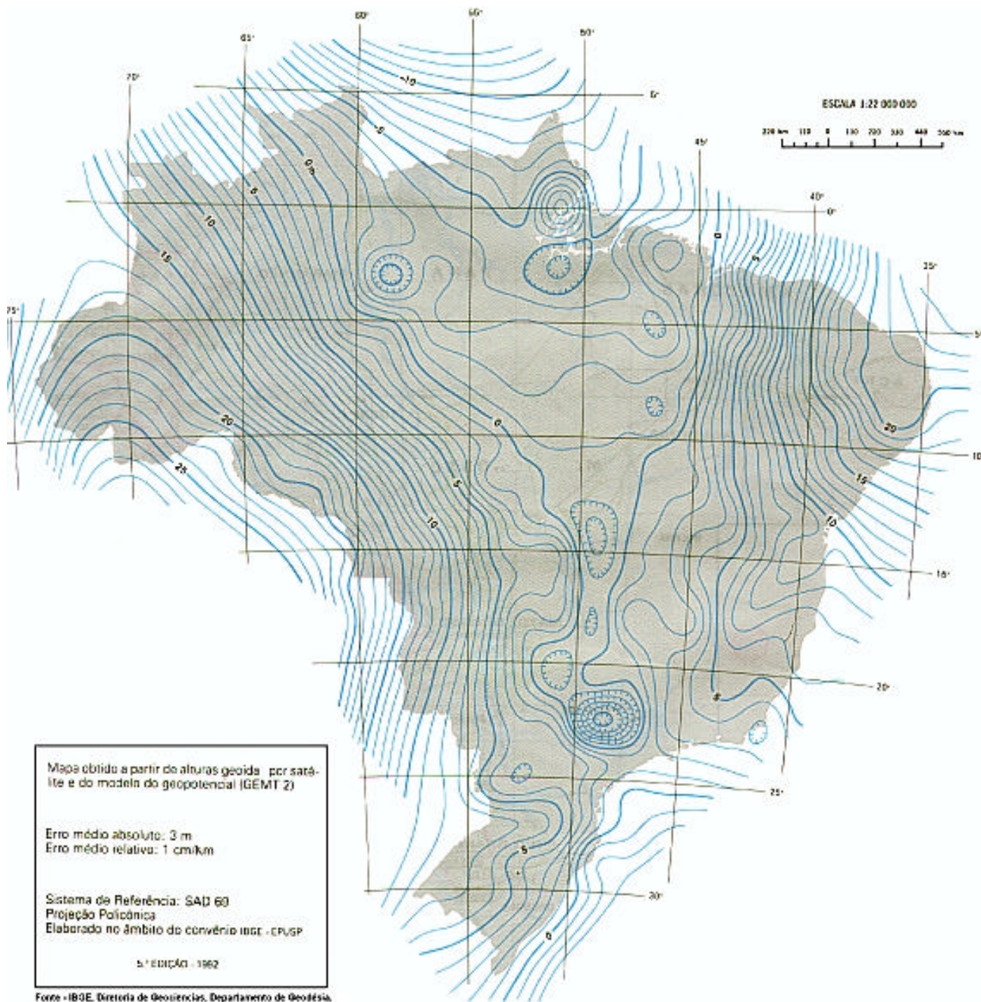
Mapa 1.6 Geoidal
